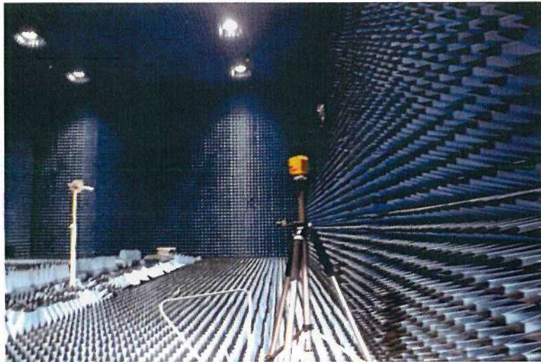
Измерительная радиобезэховая камера Государственного первичного эталона единицы напряженности электрического поля ГЭТ 45-2011
