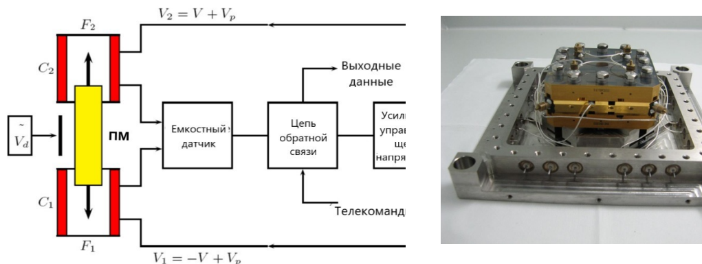
Рис. 5. Прецизионный электростатический акселерометр: схема одного канала серво-контроля акселерометра STAR [18] (слева); механическая часть прототипа акселерометра для миссии TianQin (справа)
