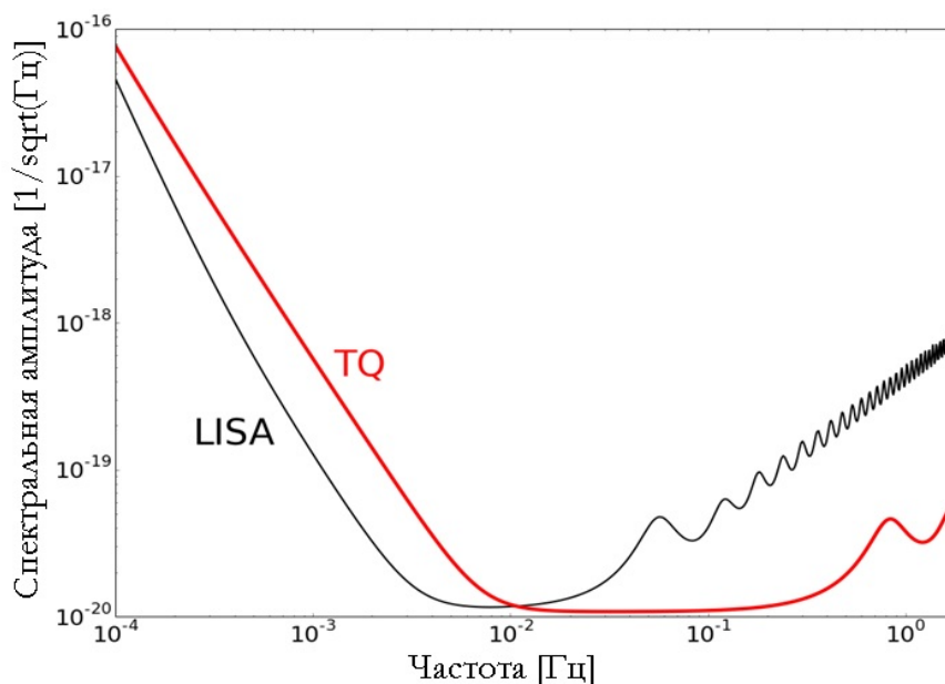
Рис. 3. Кривые чувствительности (в единицах спектральной амплитуды) проектов TianQin и LISA
