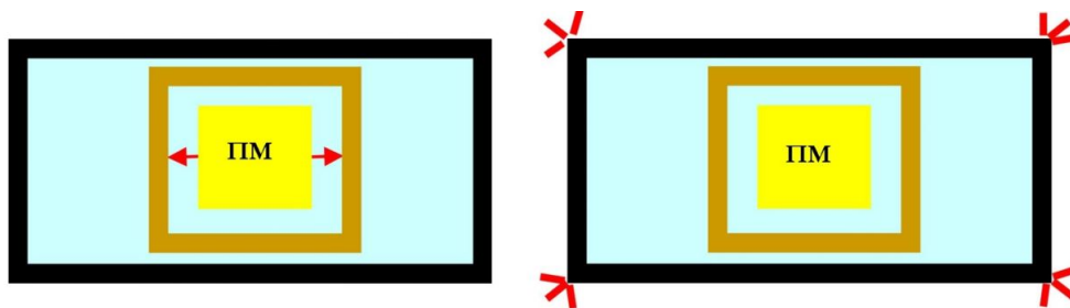
Рис. 6. Два режима работы акселерометра (пробная масса, полость акселерометра, спутник): режим измерения возмущений (слева) и режим геодезического репера (справа)
