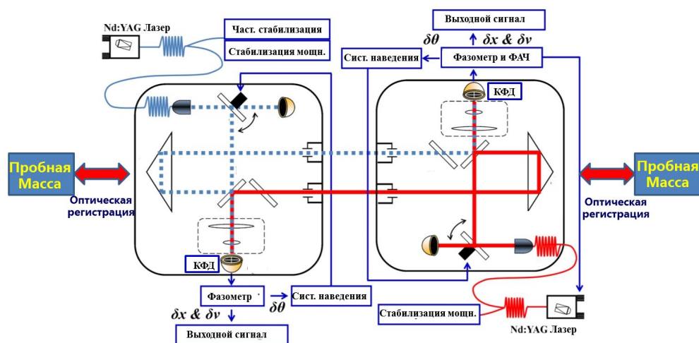
Рис. 4. Принципиальная схема межспутникового транспондерного лазерного интерферометра для детектирования гравитационных волн в космосе
