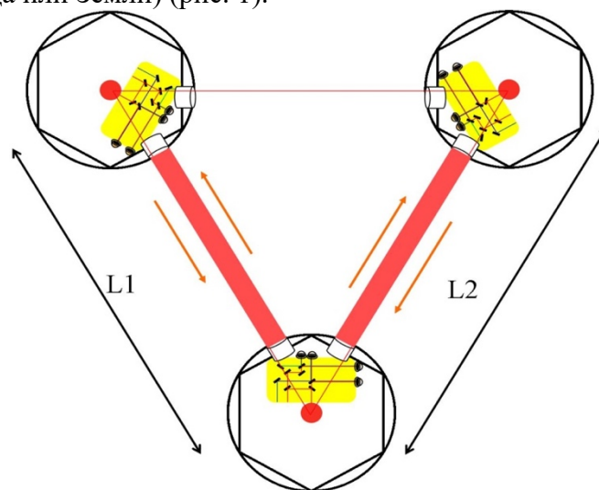
Рис. 1. Схема космического ГВ детектора. Три спутника на круговых геоцентрических орбитах. Лазерный интерферометр измеряет разность расстояний (разность фаз) между двумя плечами интерферометра, которая содержит информацию о гравитационных волнах
